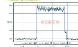
5次諧波電流趨勢圖
