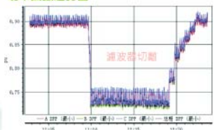
功率因數趨勢圖
