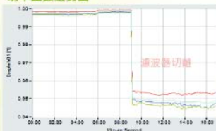
功率因數趨勢圖
